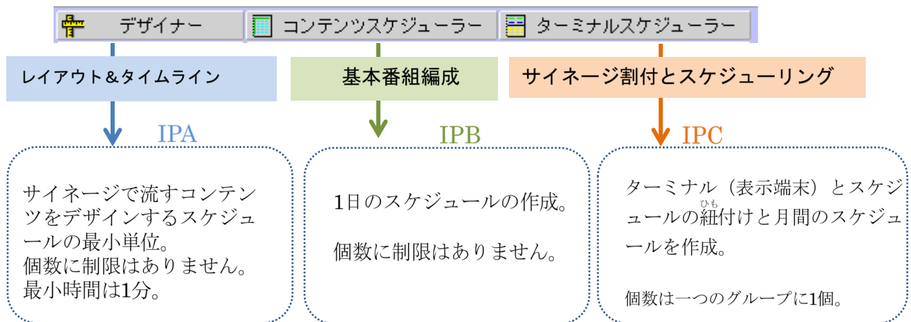
IP_STUDIO IVの設計とファイル構成
